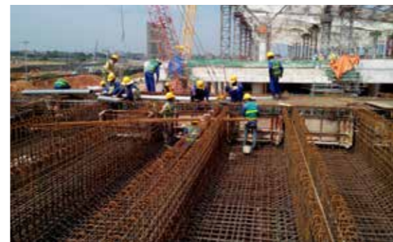
Thi công dầm cầu dẫn nhà ga T2 Nội Bài
